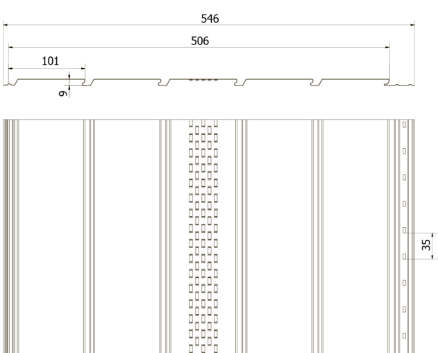
Вентиляционный (перфорированный) софит
